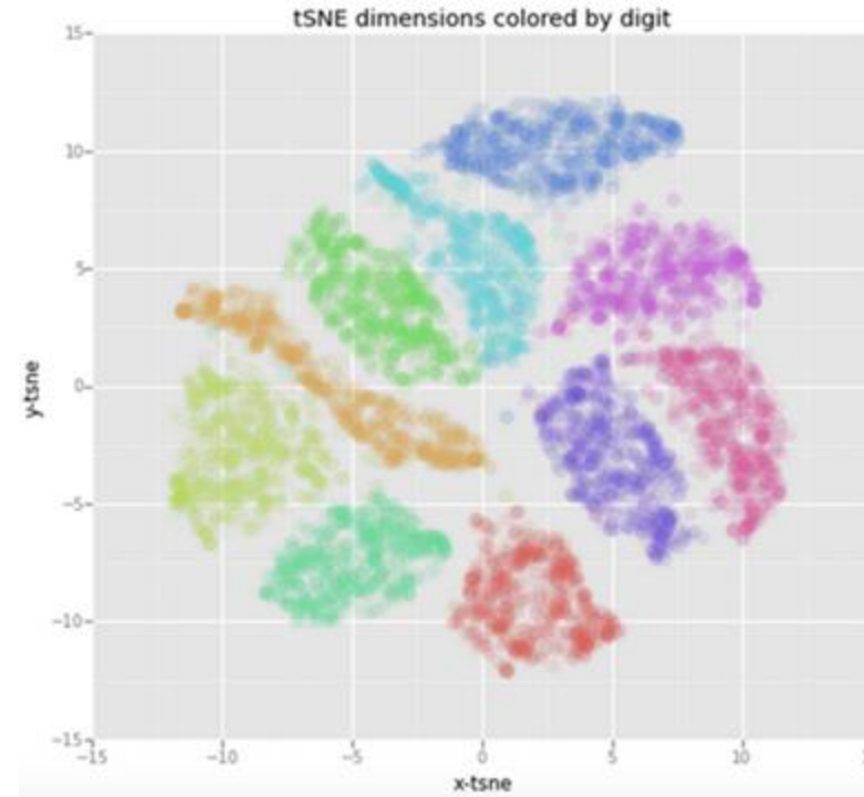
T-SNE
